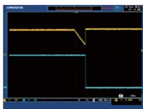
Rzeczywiste przebiegi (Kanał 1: Napięcie urządzenia testowanego Kanał 2: Prąd urządzenia testowanego)
